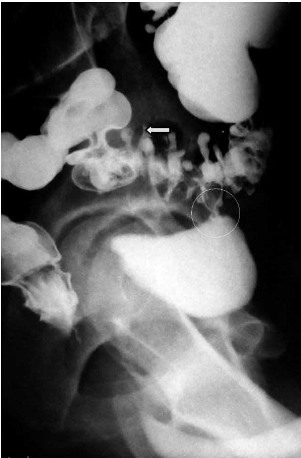
Fig. 3 - Fistola colo-vescicale.
